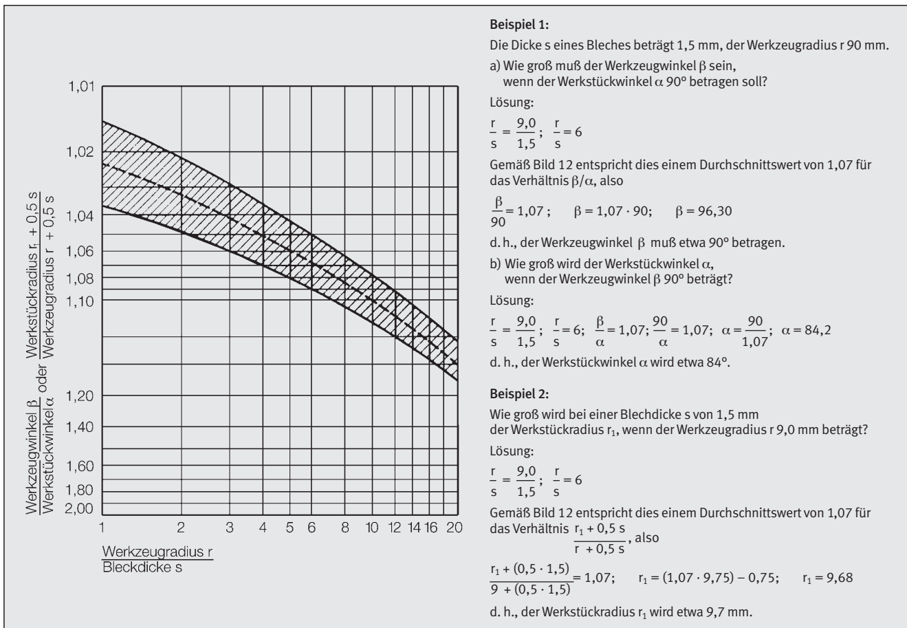
Bild 13: Beziehungen zwischen Werkzeugradius, Werkzeugwinkel, Radius und Winkel am Werkstück sowie Dicke des Materials beim Biegen weichgeglühter Bleche aus Edelstahl rostfrei
