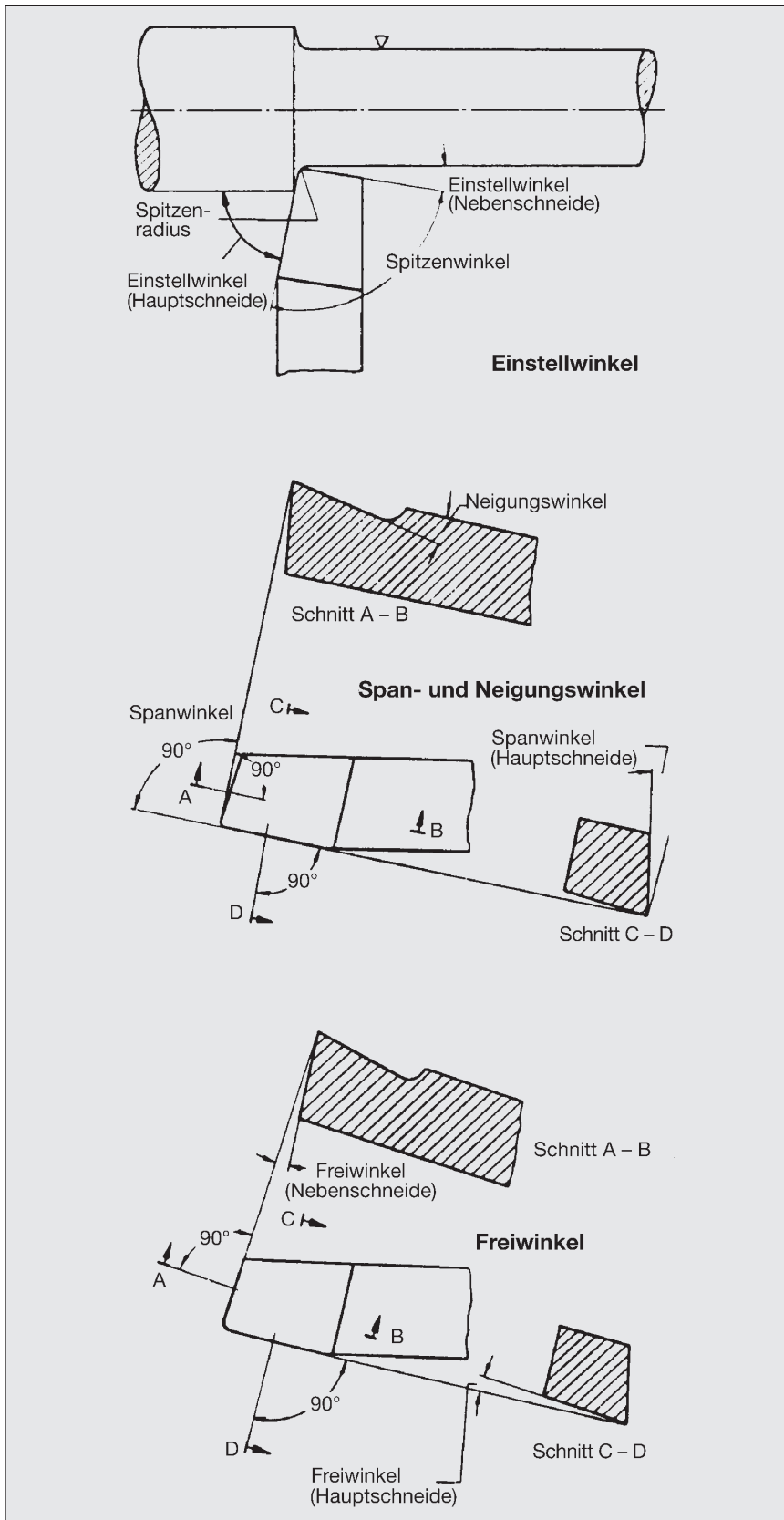
Bild 10: Drehmeißel für das Bearbeiten von Edelstahl Rostfrei: Die Schnittkante ist gerade und hat einen Einstellwinkel von 70°
