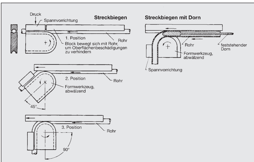
Bild 16: Das Streckbiegen von Rohren kann mit und ohne Dorn erfolgen
