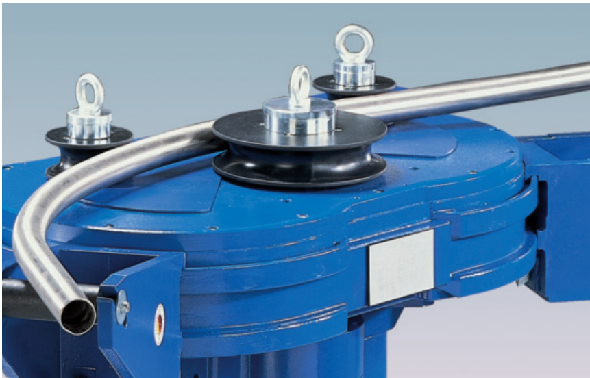
Bilder 14 + 15: Mit Walzenbiegemaschinen lassen sich Rohre aller Art in den unterschiedlichsten Radien umformen
