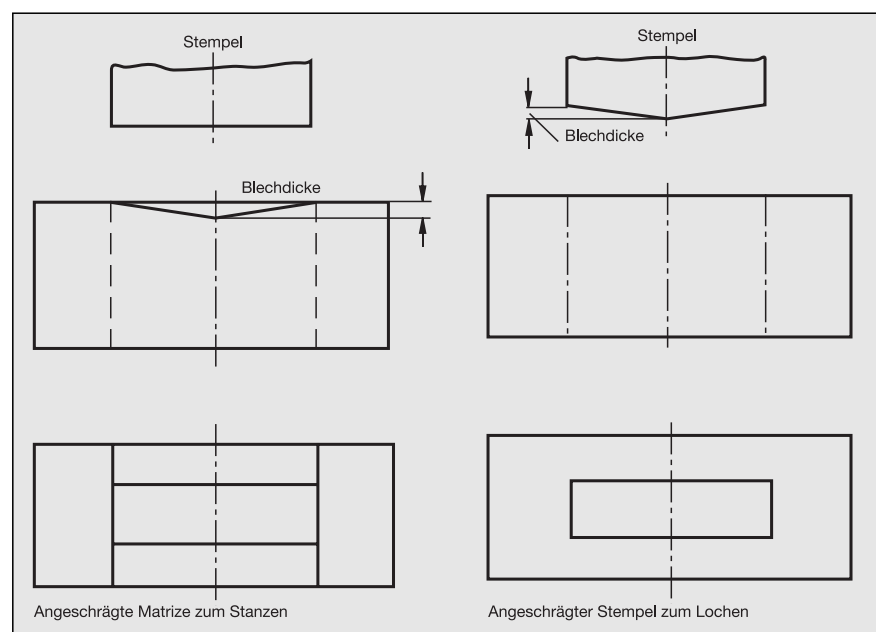
Bild 1: Darstellung der empfohlenen Werkzeugformen für das Stanzen und Lochen flacher Teile aus Edelstahl rostfrei
